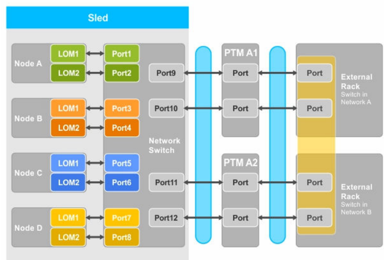
Ilustración 6. Configuración de aislamiento del adaptador de red
