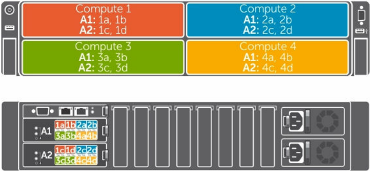
Ilustración 9. Nodo para asignación de puertos de los módulos de paso a través para la configuración de aislamiento de red mejorada
