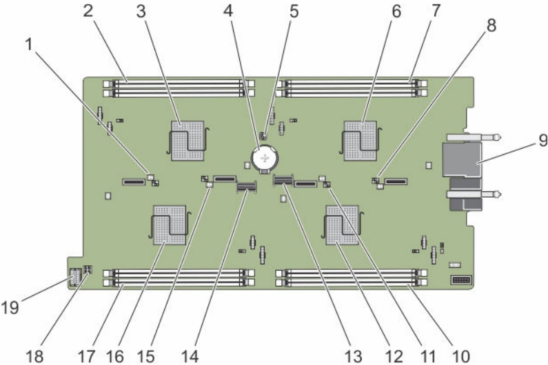
Ilustración 31. Conectores de la placa base
