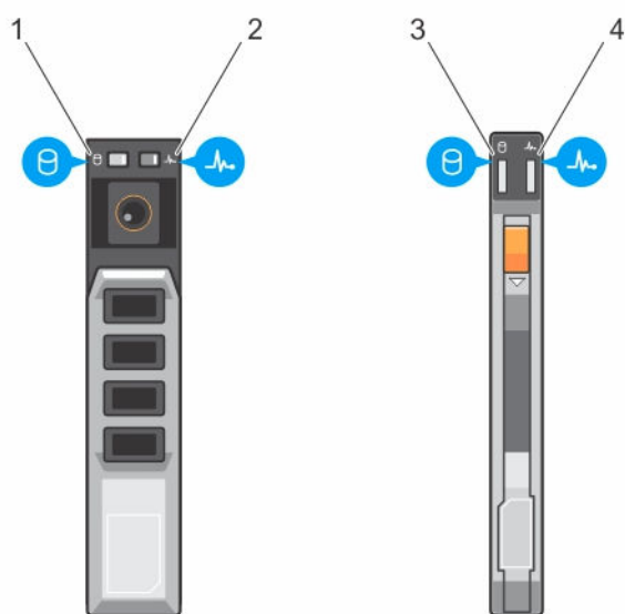
Ilustración 3. Indicadores de la unidad de disco duro/SSD
