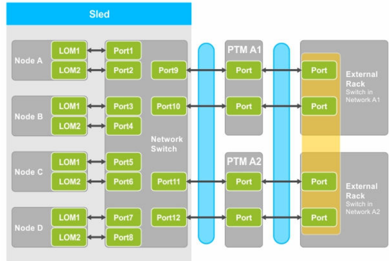
Ilustración 5. Configuración estándar
